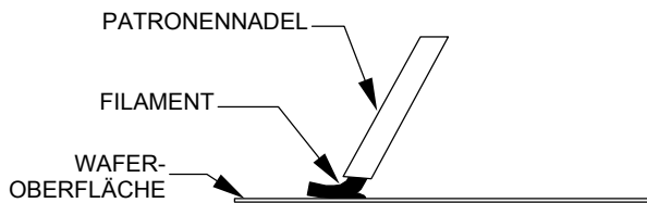
FALSCH: Filament zu dicht am Wafer
